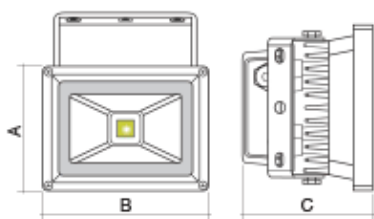
DIMENSIONES (mm)
